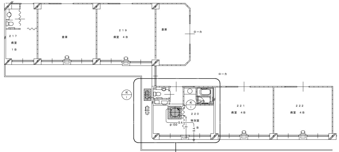
2階平面図(撤去)
